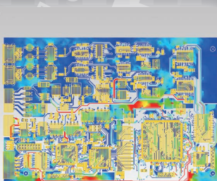
基板部分の電流分布
