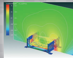
近傍電界分布
