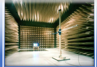
大型機械も試験可能な10m電波暗室
