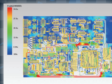
基板部分の電流分布
